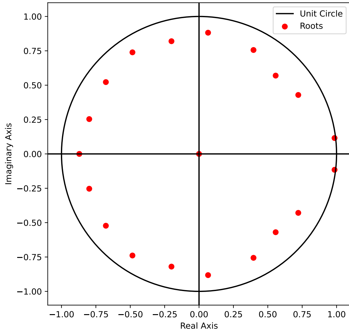
L1 AR(20) roots
